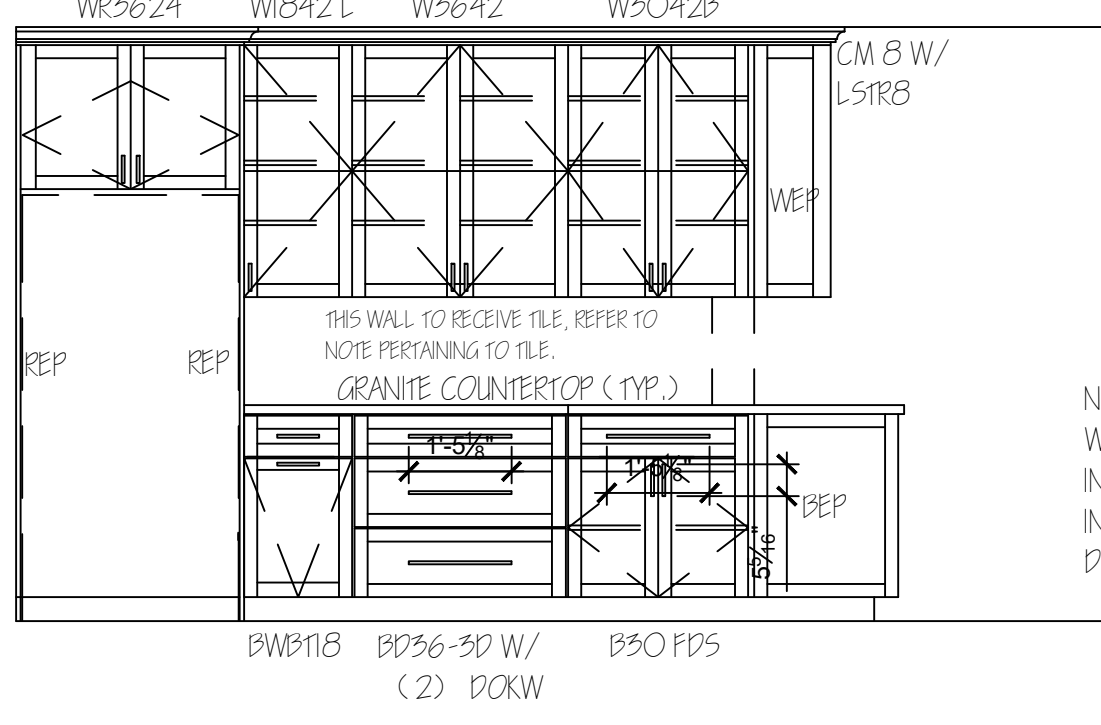
ELEVATION 3a/ A-101
