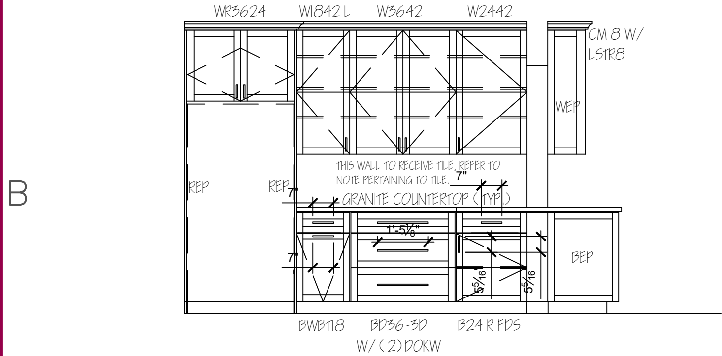
ELEVATION 3/ A-101
