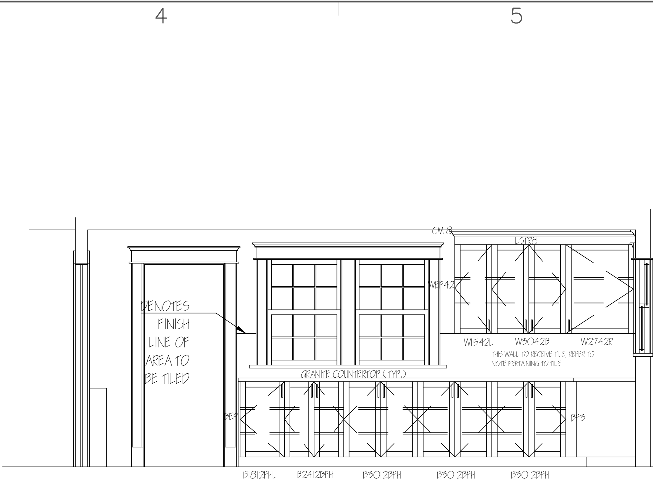
ELEVATION 1/ A-102
