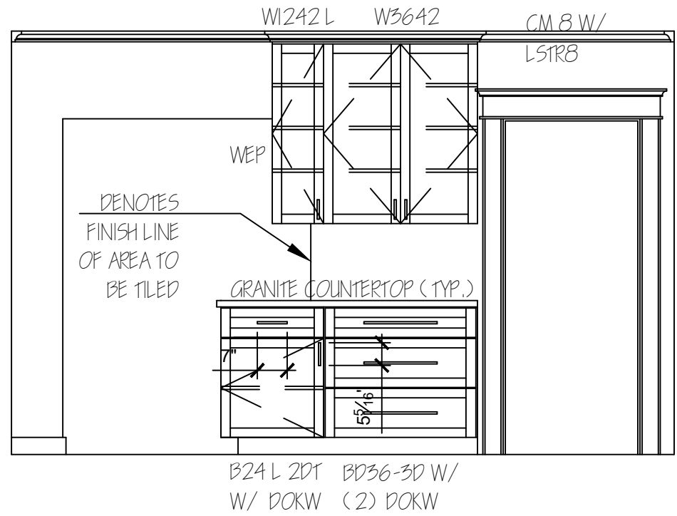
ELEVATION 4/ A-101
