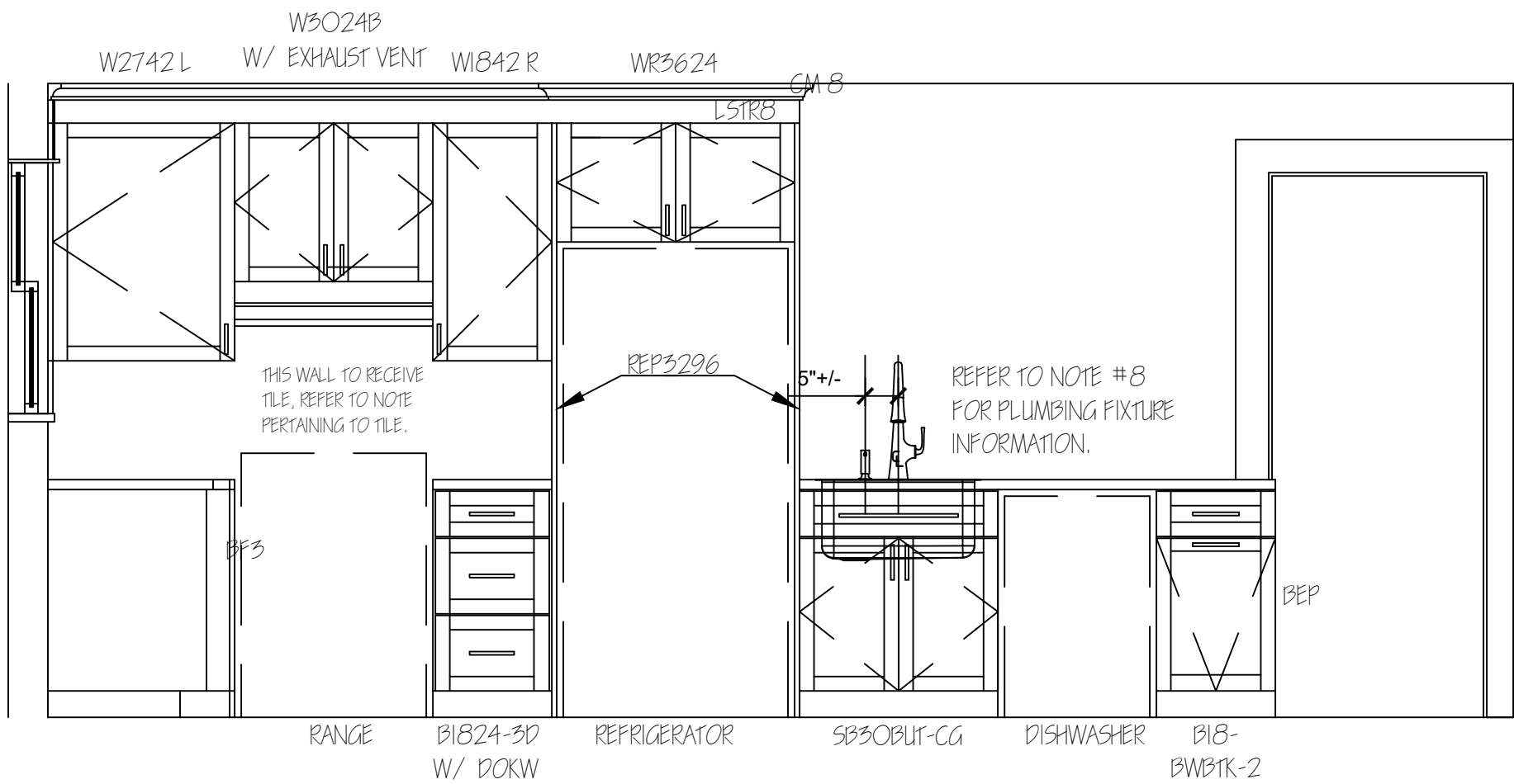
ELEVATION 3/ A-102
