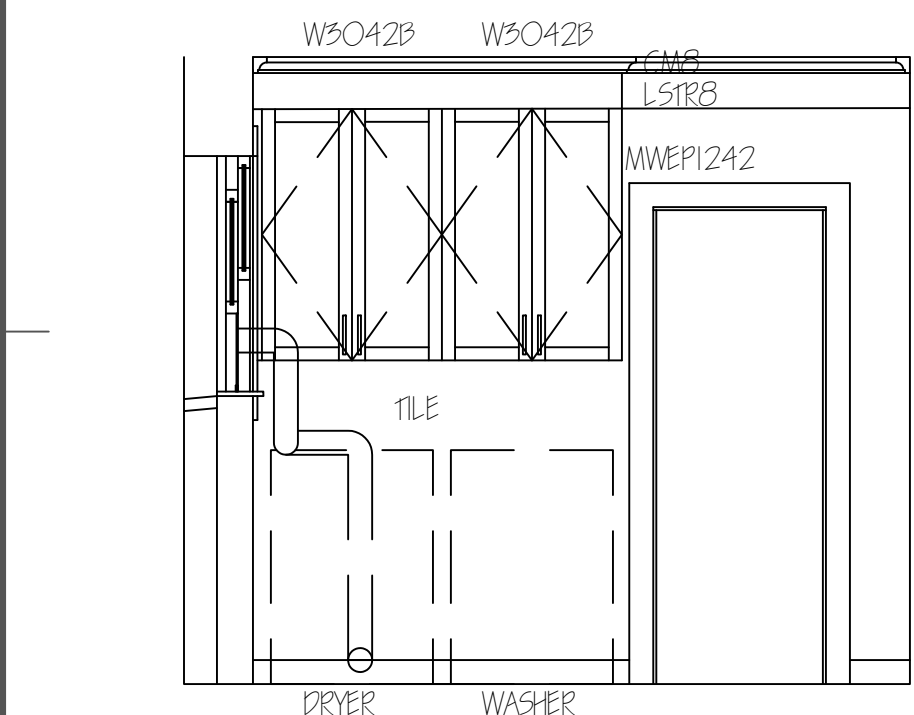
ELEV. 6/ A-100
