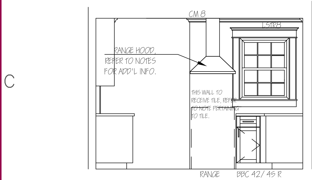
ELEVATION 2/ A-101
