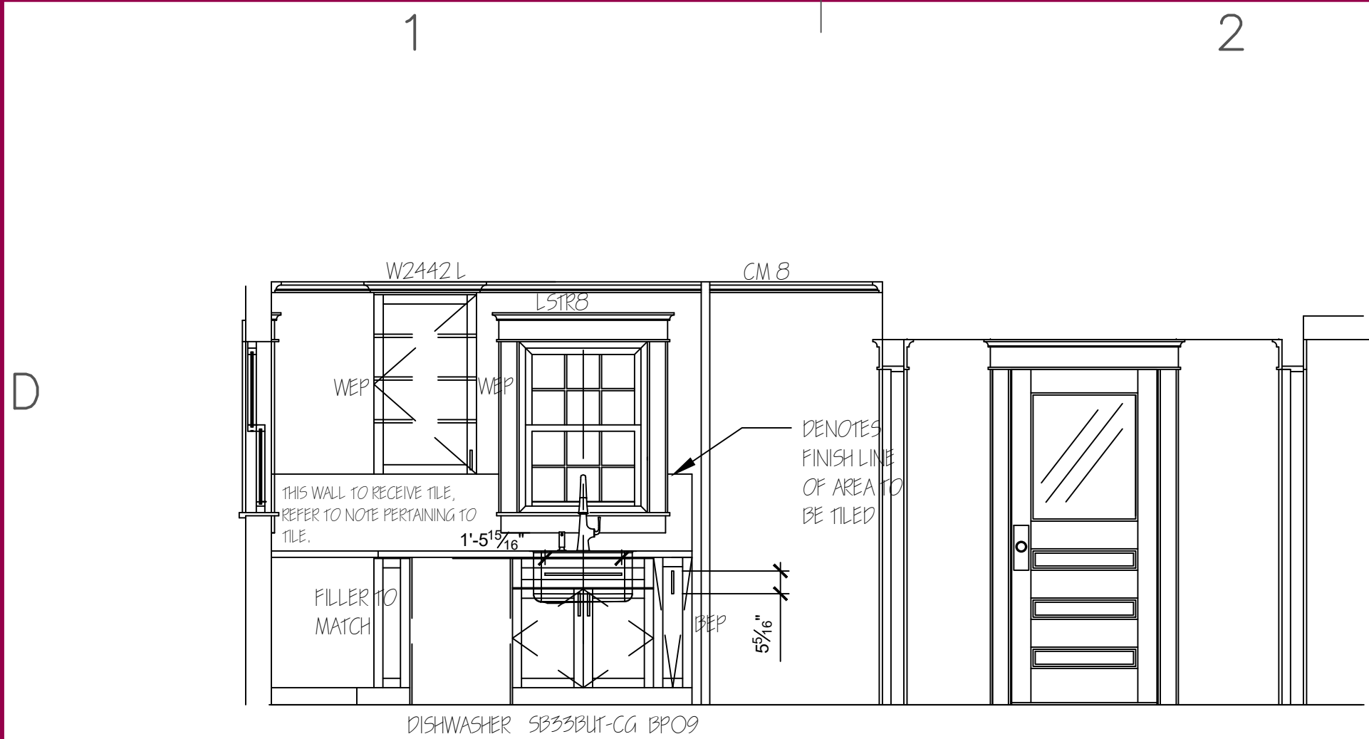
ELEVATION 1/ A-101
