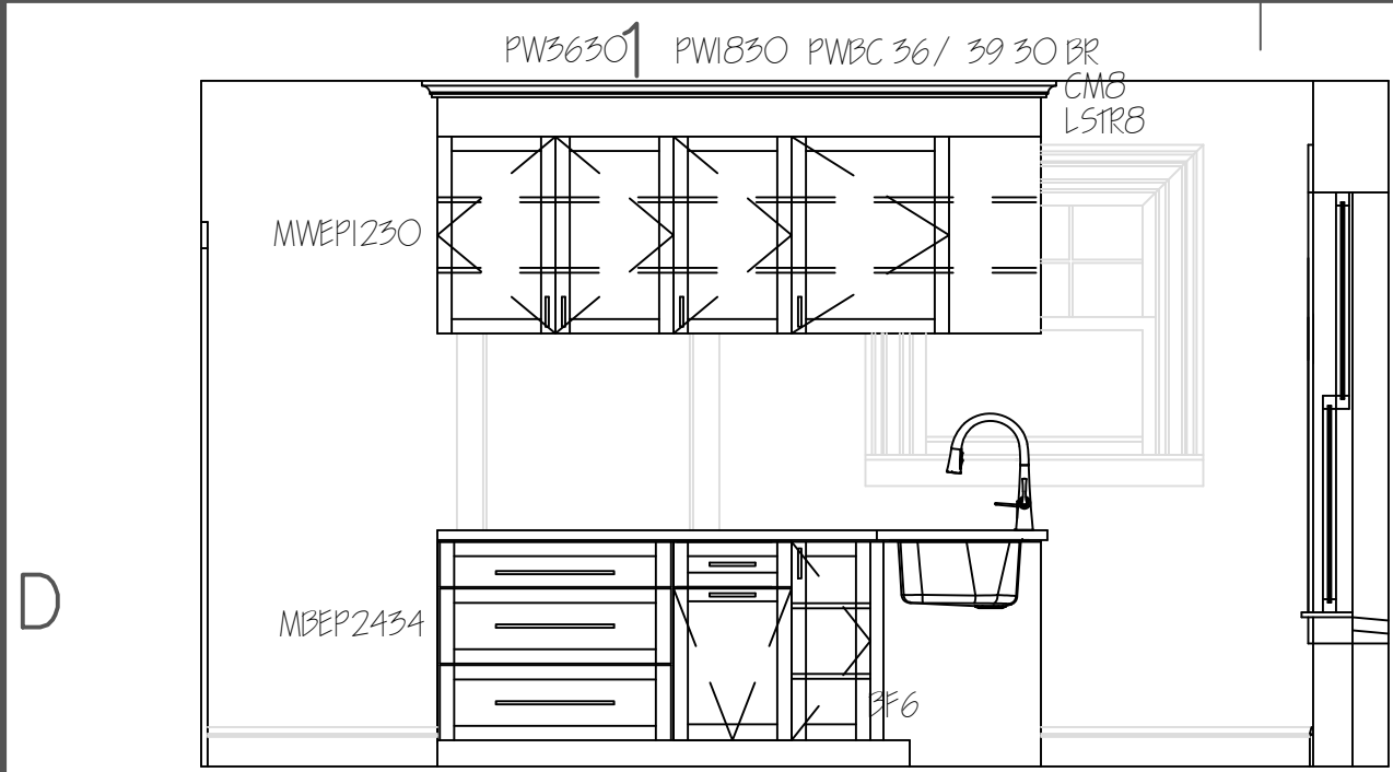
ELEVATION 1/ A-100
