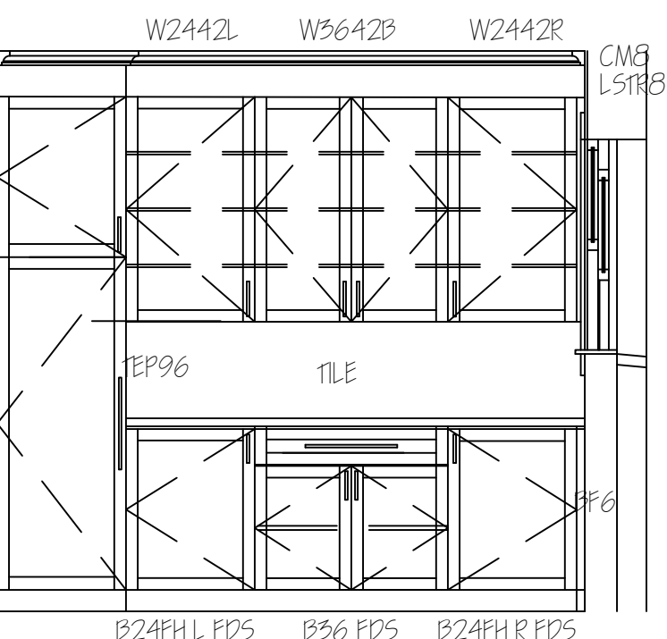
ELEV. 7/ A-100
