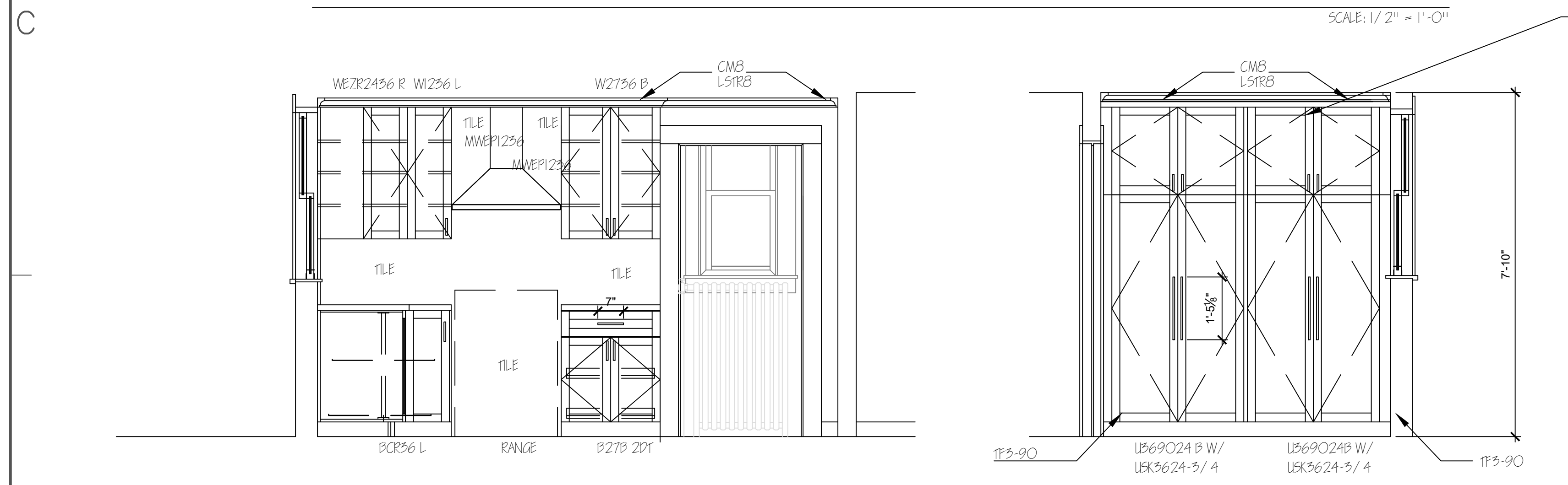
ELEVATION 2 / A-100
