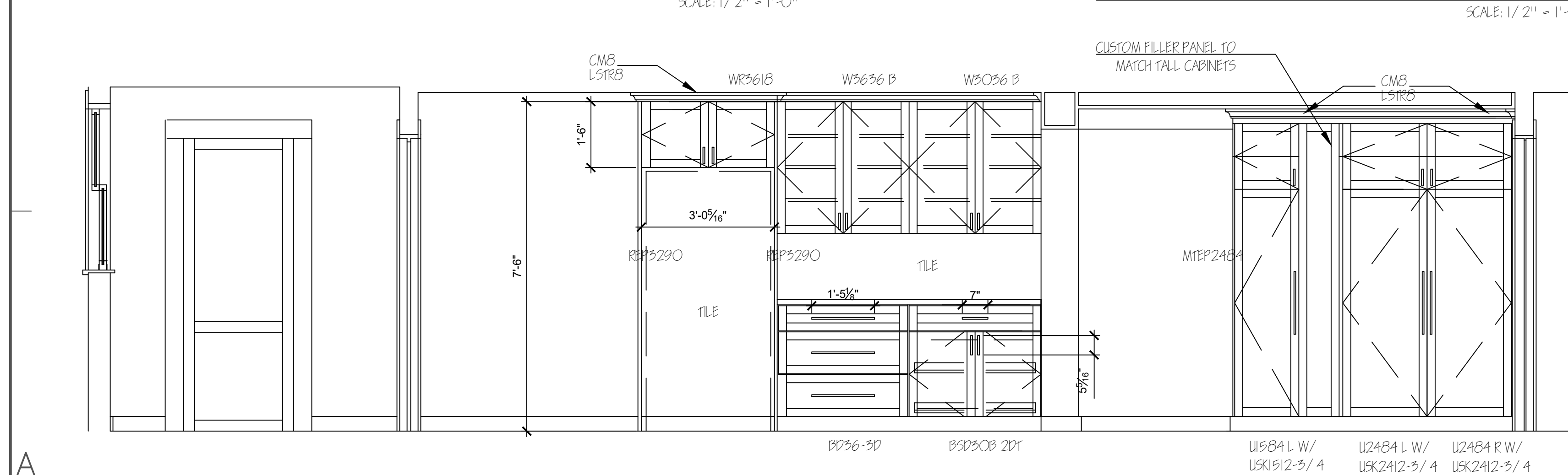
ELEVATION 4 / A-100
