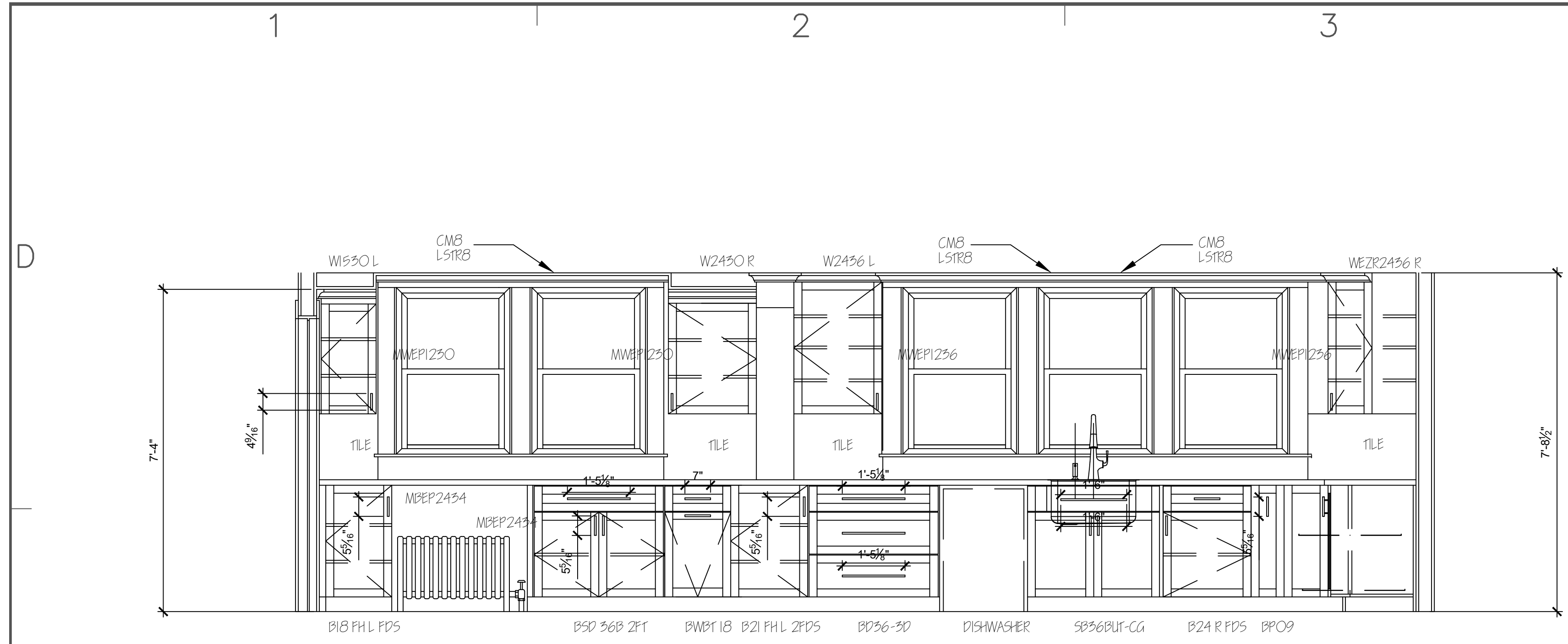
ELEVATION 1 / A-100
