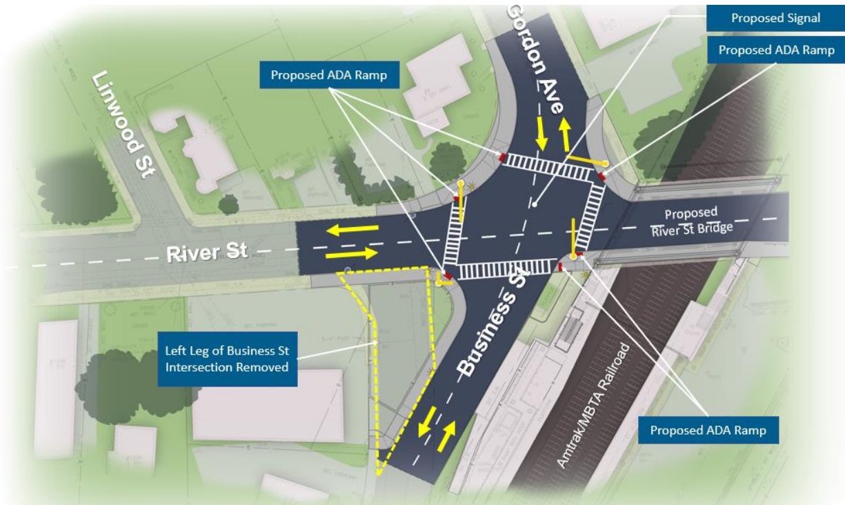
Fig 5: Amelyorasyon yo pwopoze pou entèseksyon West Street/Business Street/Gordon Avenue
