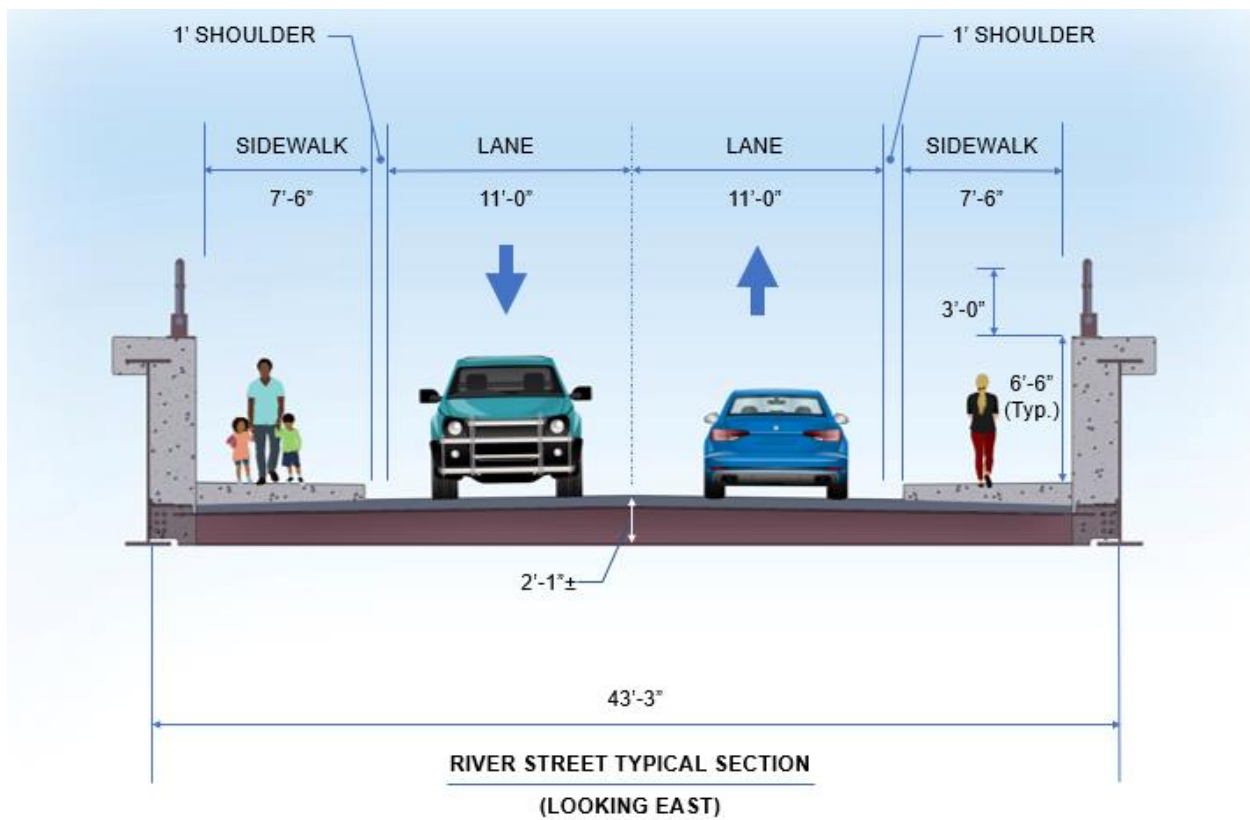
Fig 2: Koup transvèsal Pwojè yo pwopoze pou ranplasman pon an
