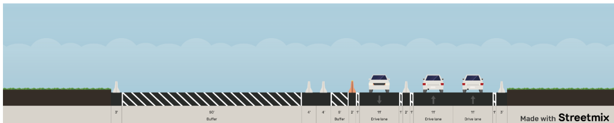
Figura 3: Configuración del tráfico prevista actualmente para el período de construcción en la I-391
