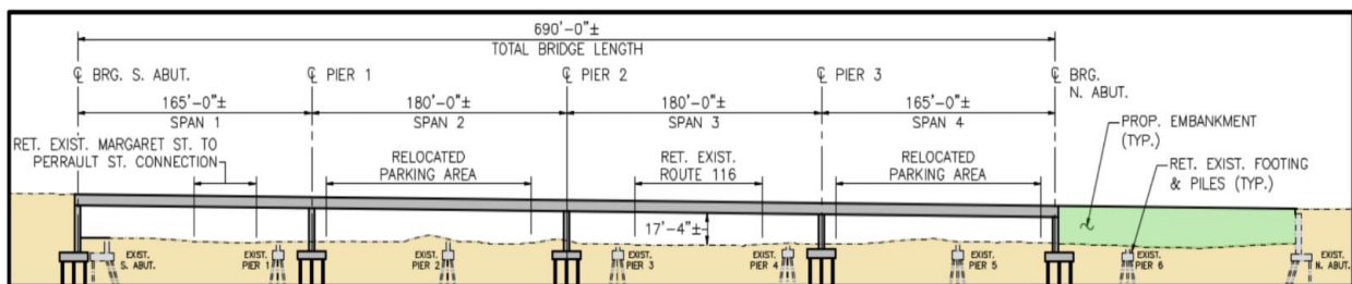
Figura 2: Configuración del puente de reemplazo prevista actualmente
