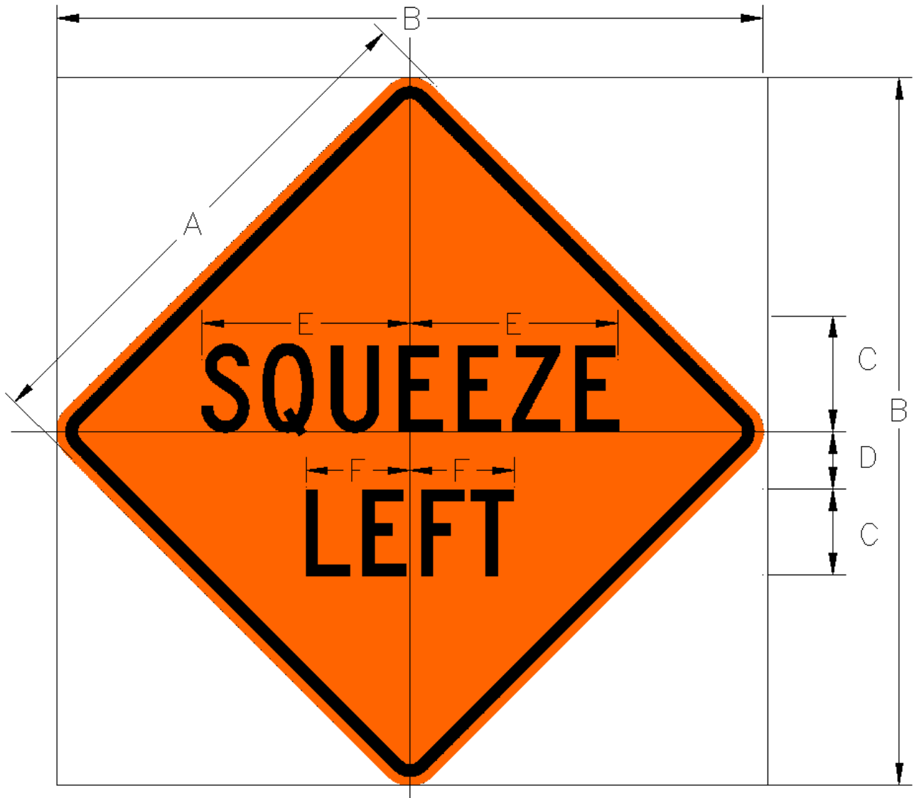
MA-W30-8L SQUEEZE LEFT
